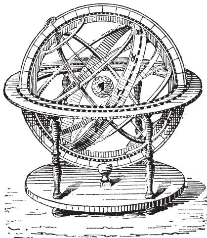
Рис. 3. Модель небесной сферы
