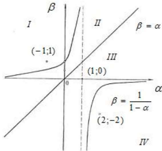
Рис. 8.2. Плоскость параметров (\alpha, \beta)
