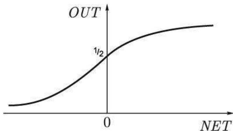
Рис. 15 – Сигмоидальная (S-образная) функция
