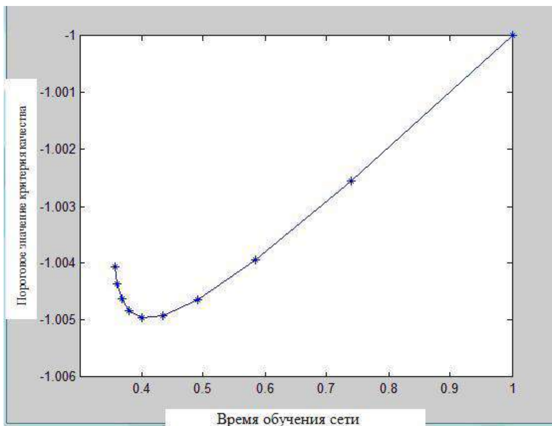
Рис. 22 – График обучения нейронной сети
