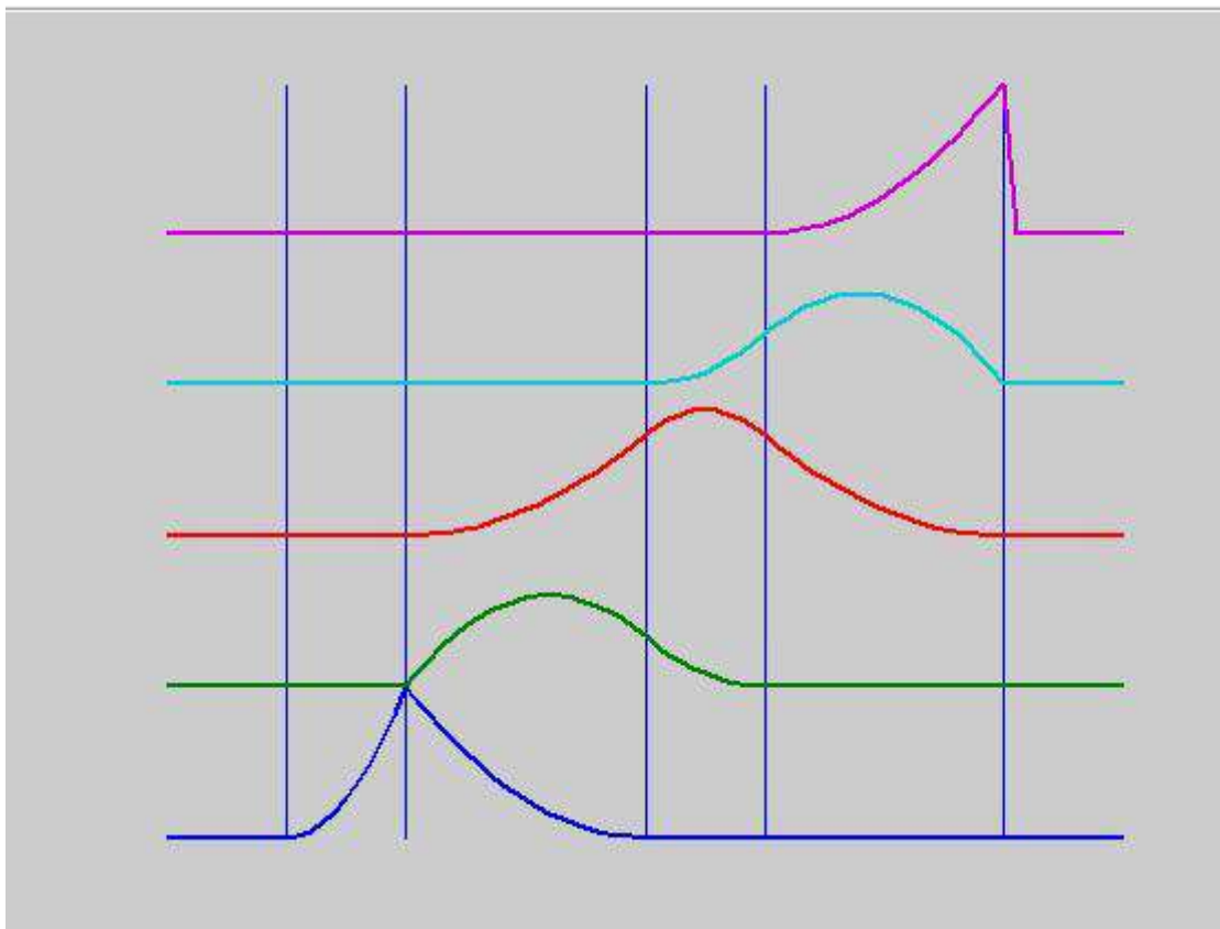
Рис. 8 – Сплайновая аппроксимация
