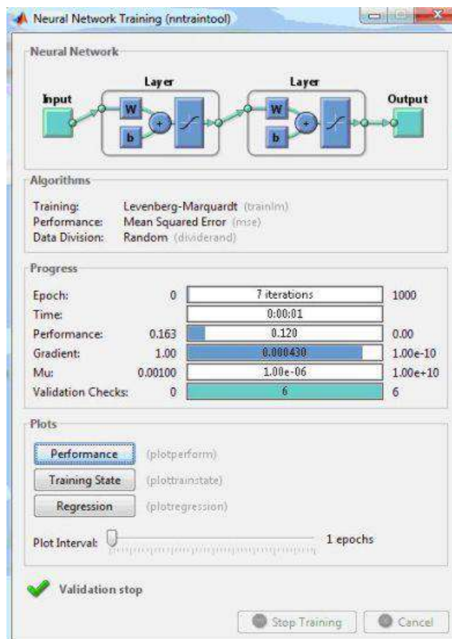
Рис. 28 – Результаты обучения
