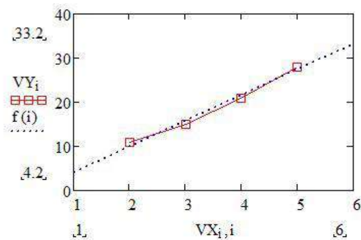
Рис. 3 – Линейная регрессия
