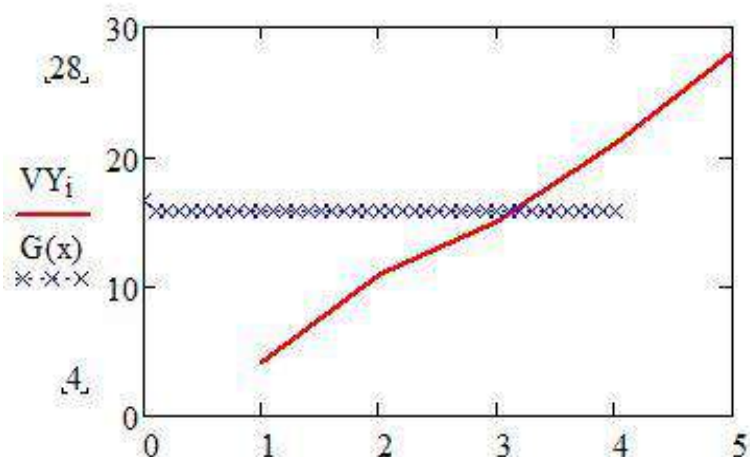
Рис. 6 – Регрессия нелинейная общего вида
