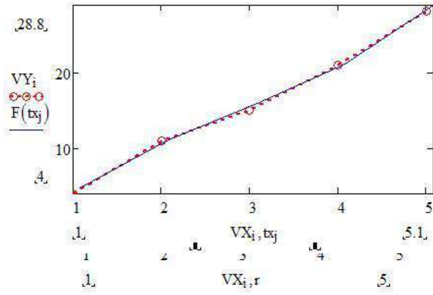
Рис. 5 – Полиномиальная регрессия
