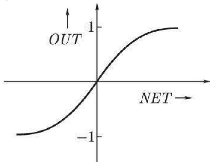
Рис. 16 – Гиперболический тангенс
