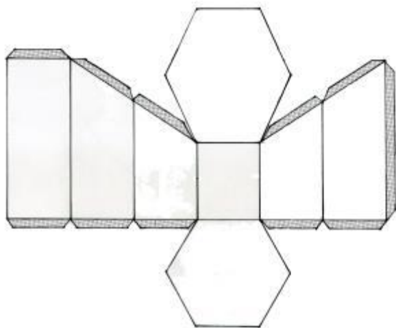
Рис. 121. Развертка усеченной призмы с шестиугольным основанием
