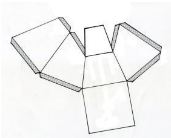
Рис. 137. Развертка усеченной пирамиды с квадратным основанием
