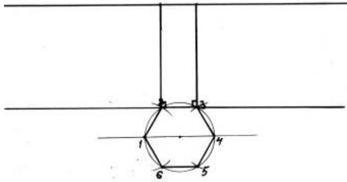
Рис. 81. Построение грани боковой поверхности призмы
