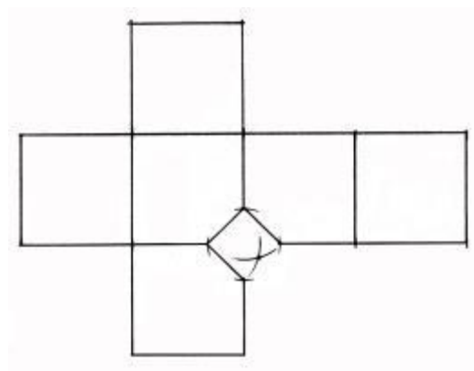
Рис. 114. Определение вершины фигуры сечения
