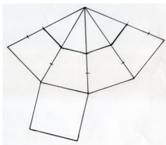
Рис. 124. Построение боковой поверхности усеченной пирамиды
