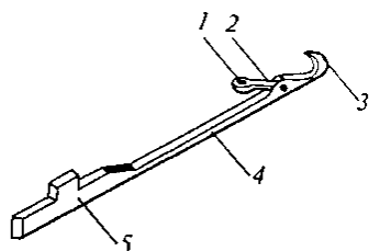
Рис. 1.32. Язычковая игла: 1 – чаша; 2 – язычок; 3 – крючок; 4 – стержень; 5 – пятка
