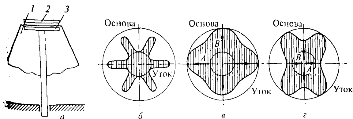
a – схема прибора: 1 – проба; 2, 3 – диски; b – d – проекции проб
